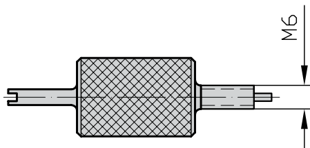
Vorrichtung für Ventil (Ablassen und Ausbau) Valve device (unloading and extraction)
